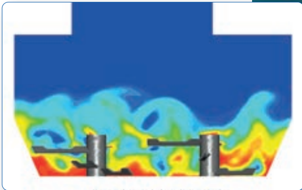
高端模拟型砂浓度（内部剖面图）
